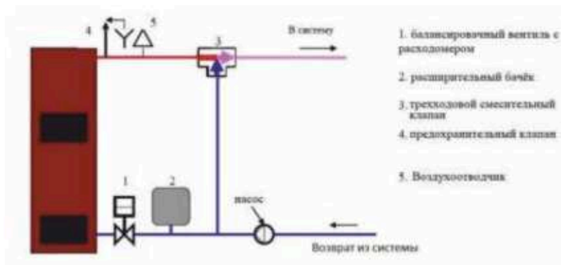
Схема подключения котла. Рисунок 8
