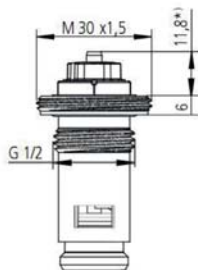
*) Клапан закрыт
